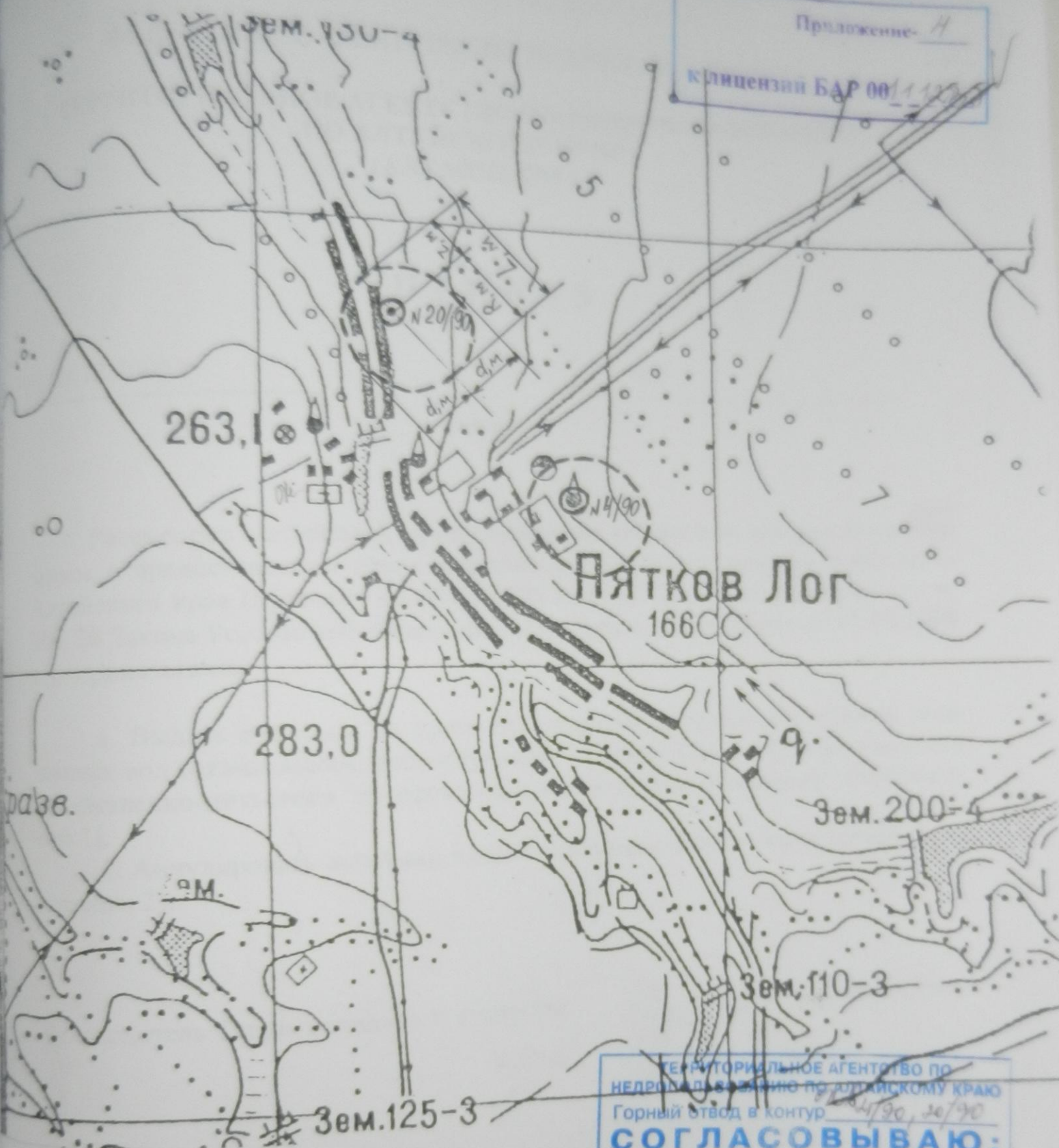
Рис. 1. ЗСО водозабора подземных вод Масштаб 1:25000
