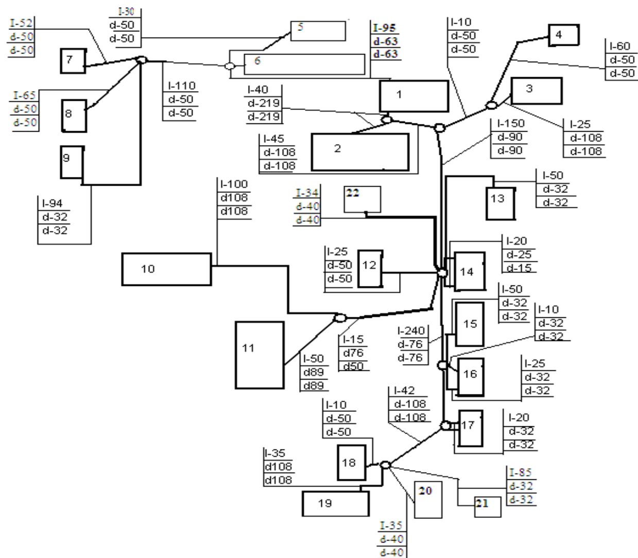
Схема сетей теплоснабжения котельной № 3
