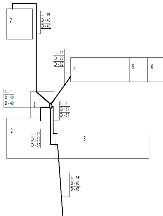
Схема сетей теплоснабжения от котельной № 4 (часть 3)
