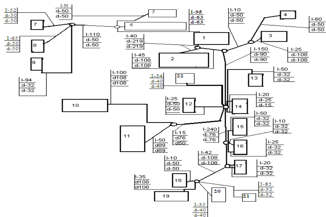
Схема сетей теплоснабжения котельной № 3 с. Волчиха, ул. Советская, 118 к
